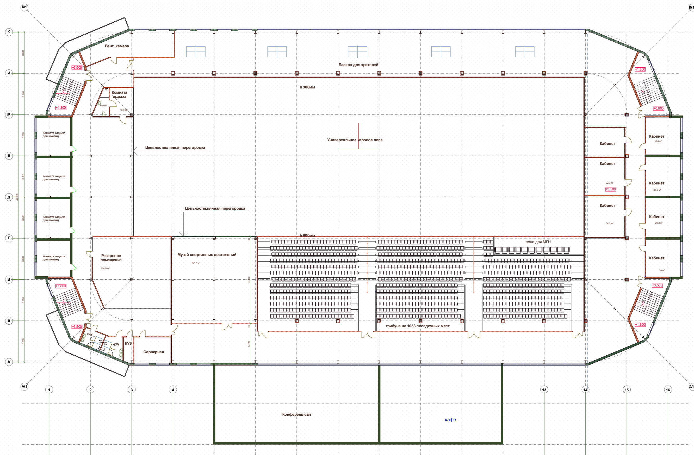
План 2-го этажа
